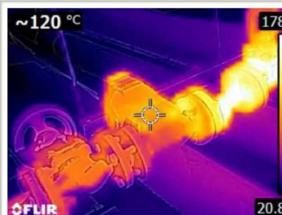
Image thermique
